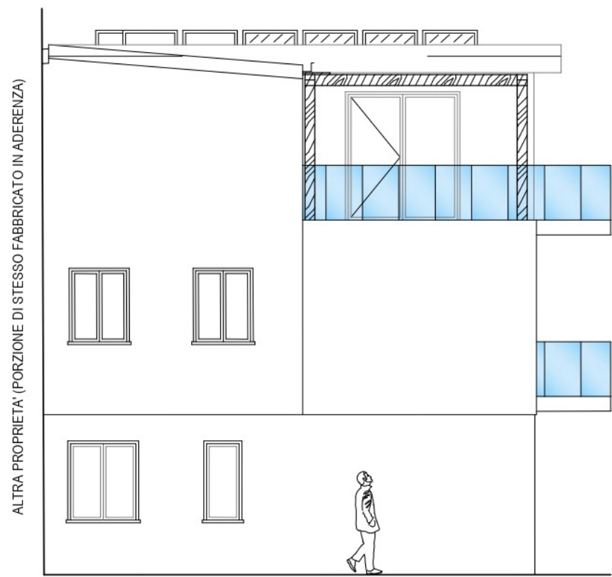
PROSPETTO SUD
